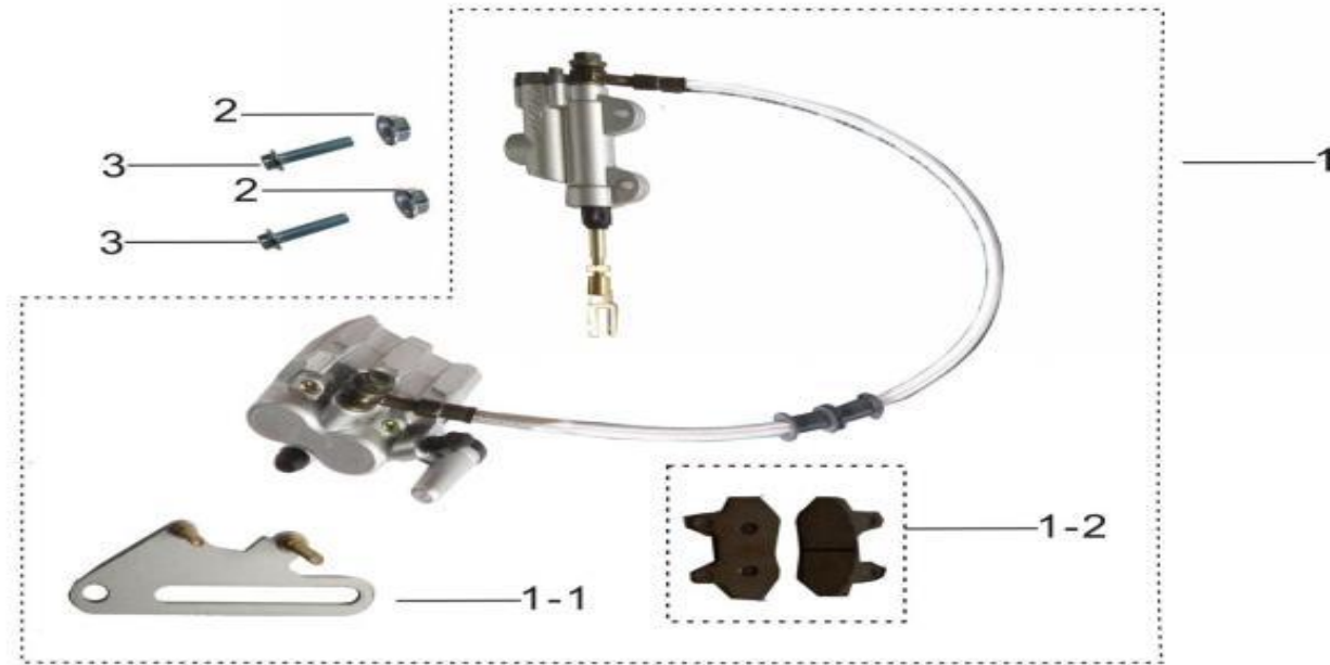
后制动总成
